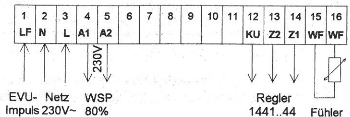
Bild 7: Anschlußschema Typ 1466/69
