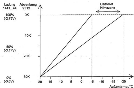
Bild 5: Steuerkennlinie
