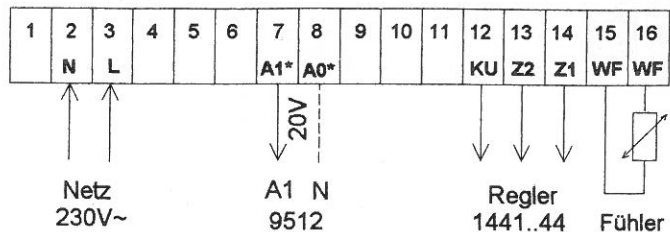
Bild 6: Anschlußschema Typ 1465/68
