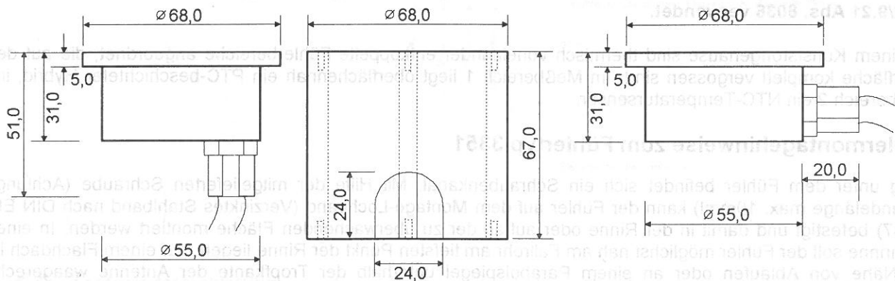
Seitenansicht Eisfühler Typ 3352
