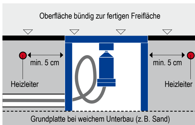
Montage mit Bodenröhre in Freiflächen
