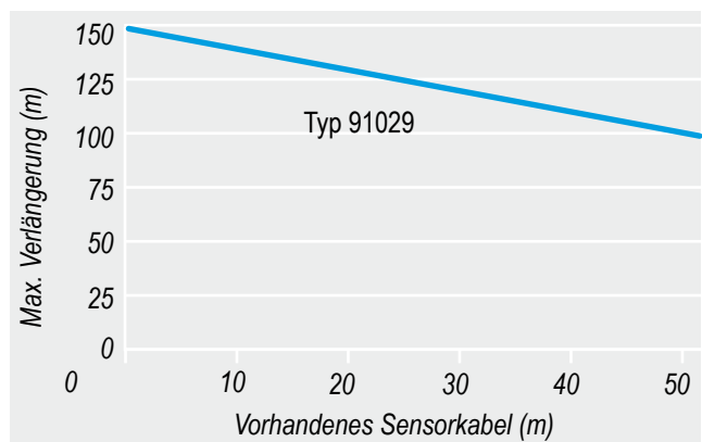
Verlängerung des Sensorkabels
